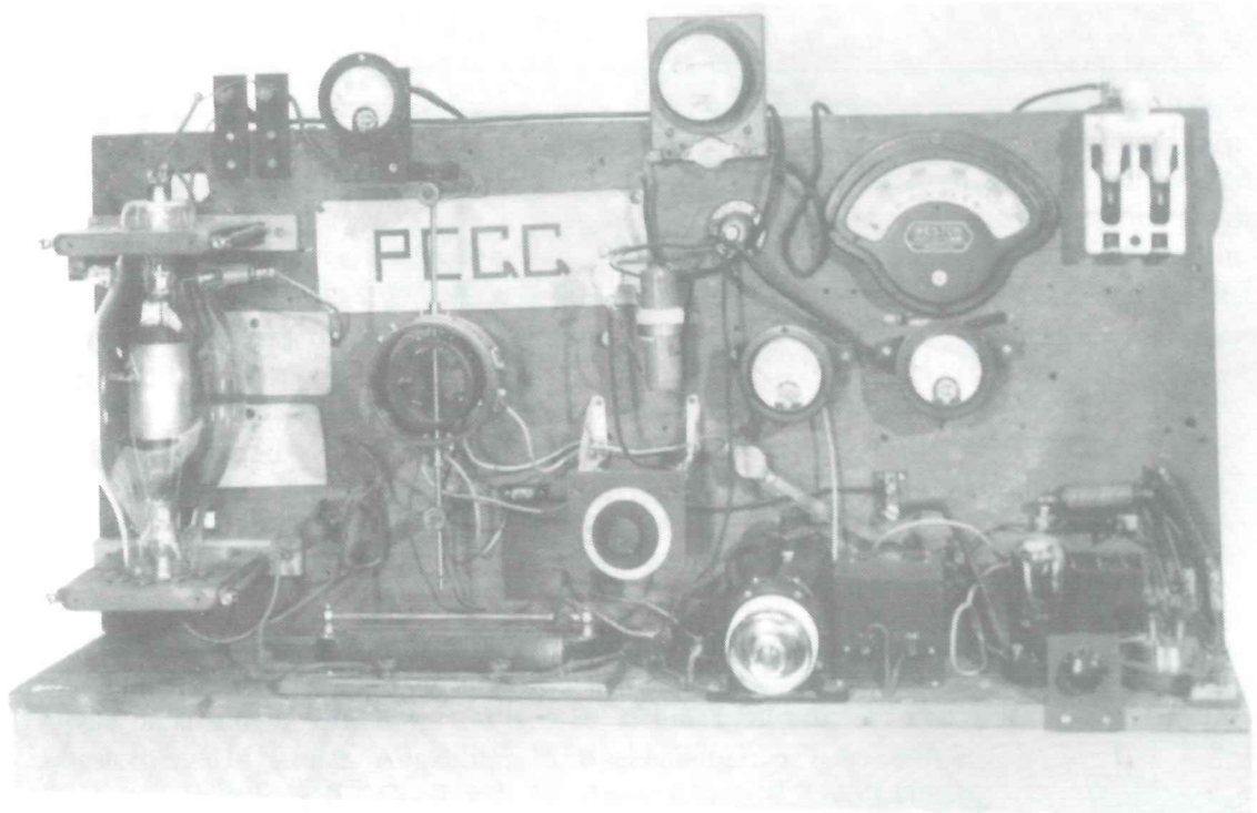
1. De beroemde experimentele zender PCGG uit 1919.
