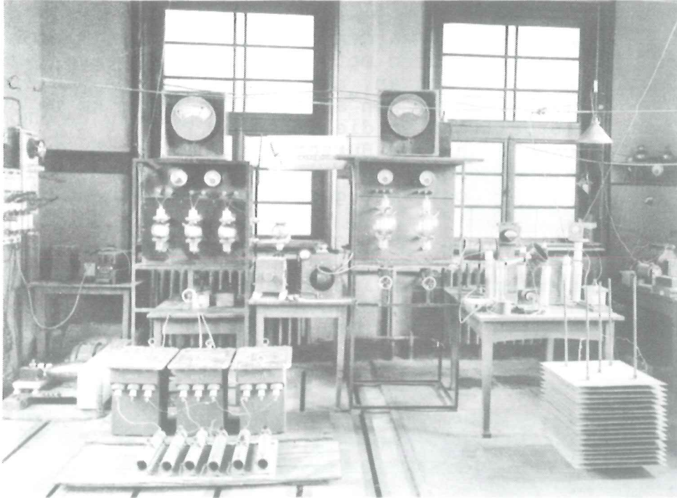
3. Laboratoriumopstelling van de eerste NSF-omroepzender, zoals die in 1923 met 500 W in de lucht kwam.
