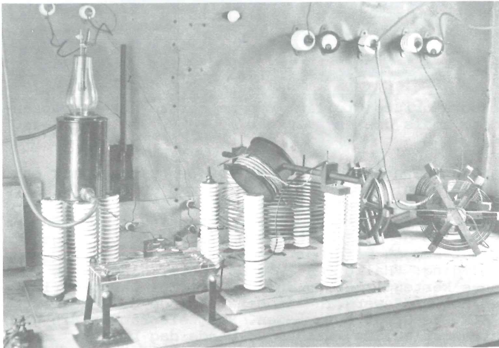
2. Een buis, wat spoelen en geloof als bouwstenen (NSF).
