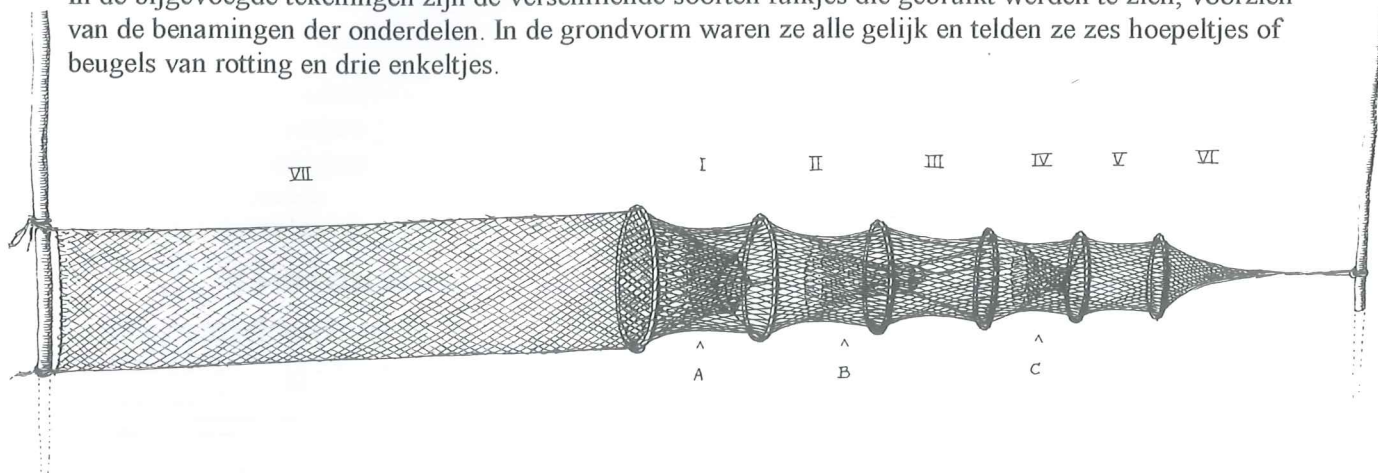
Eénvleugelige fuik. I t/m V eerste t/m vijfde rak; A, B en C eerste t/m derde enkel; VI snoet en VII vleugel.
